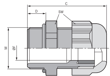
SKINTOP® KR-M ATEX plus blue
