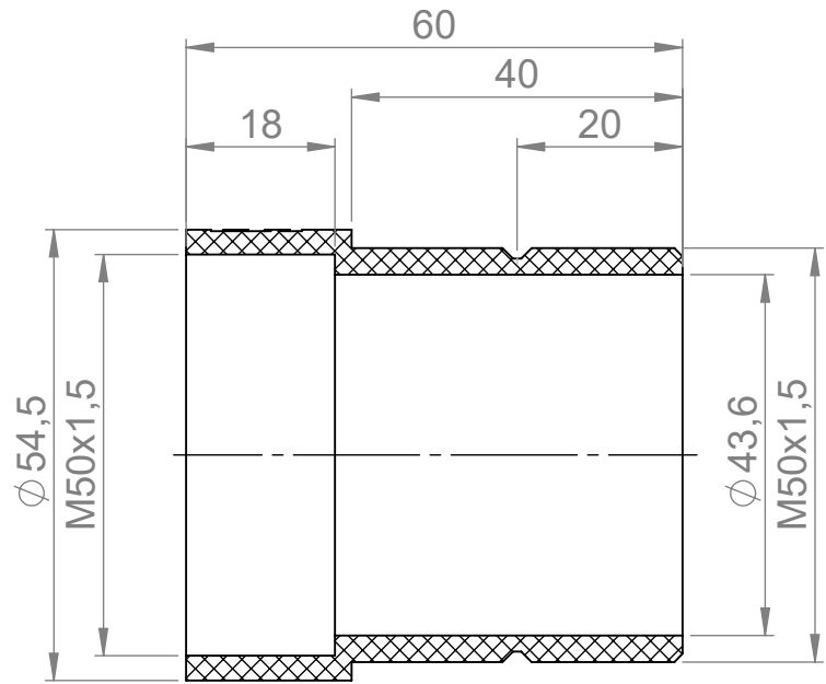
SCHNITT A-A
